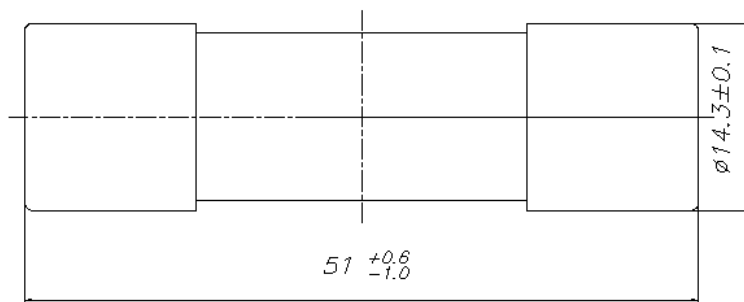
HMPV-32 DC1500V 光伏熔断体外形尺寸
