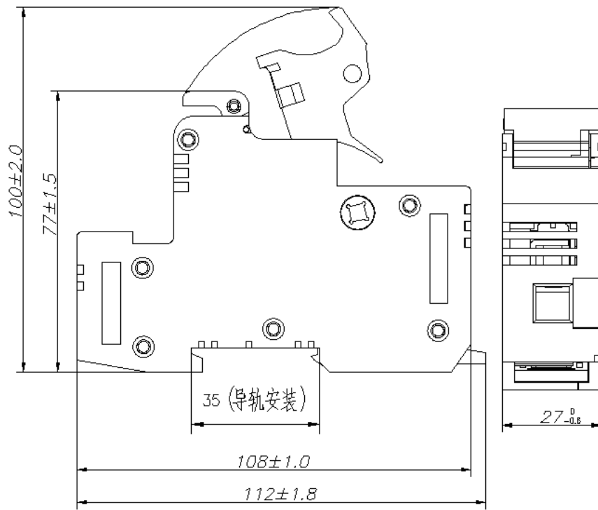
HMPV-32 DC1500V 底座外形及安装尺寸
